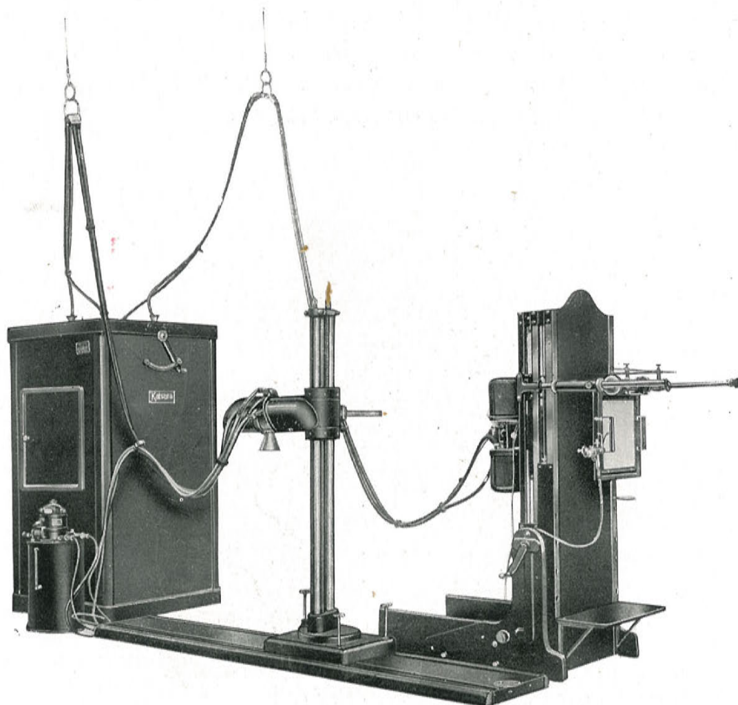
(管球二個式防電撃型)
